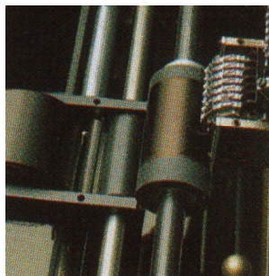
tête de numérotation et rouleau encreur microporeux
